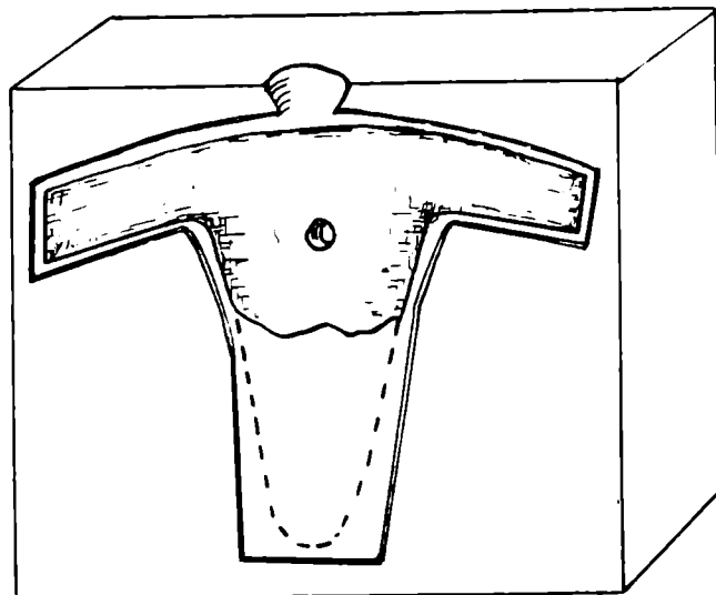
Рис. 3. Верхнебаксанский клад. Реконструкция литейной формы для рукояток кинжалов.
