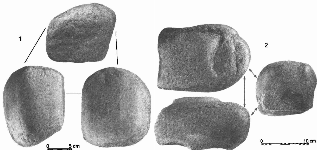
Рис. 6.15. Наковальни на валунах: 1 – кв. 4627, жертвенная яма №84 под полами плавильного двора комплекса №1, субфаза B-1 (вес 2020 гр.); 2 – кв. 3839, жилище №49, субфаза B-1 (вес 4980 гр.)
