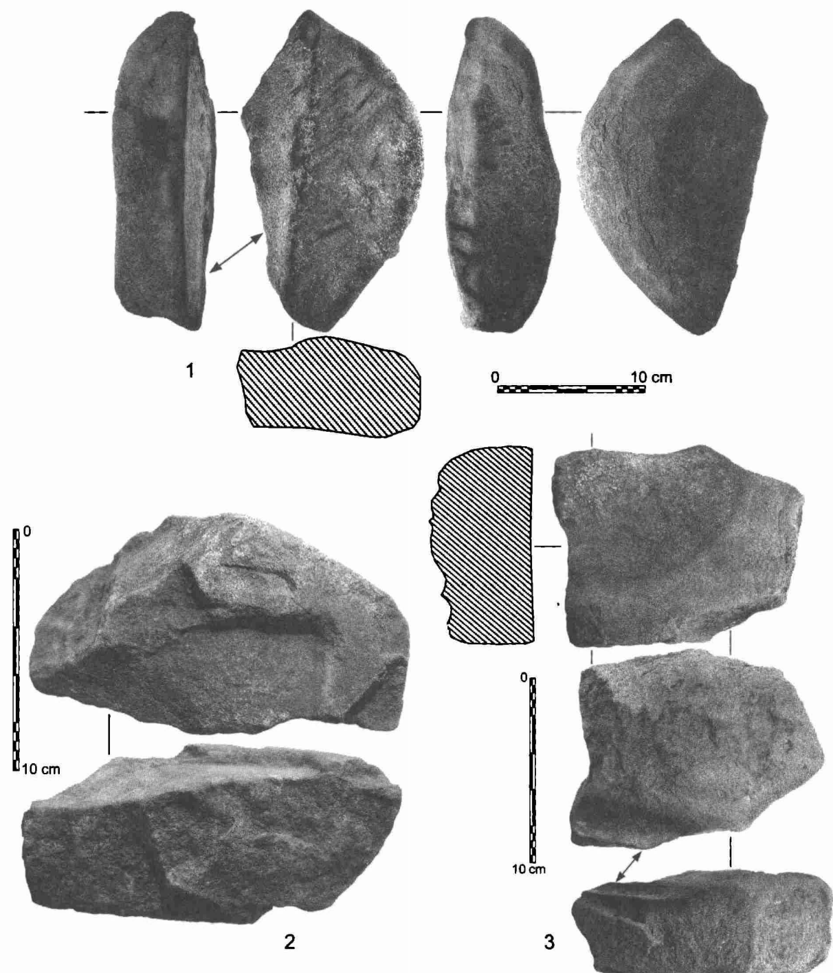
Рис. 5.3. Литейные формы: кирки-пешни; песчаник
