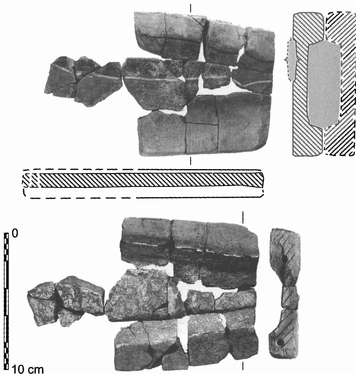
Рис. 5.10. Комплект литейных форм: клинья/тесла, ножи (кв. 5027-5028, жилой отсек комплекса №1, субфаза B-1 ); мергель
