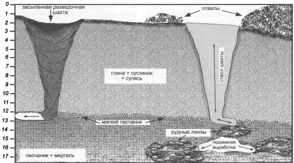
Рис. 9.6. Стратиграфическая схема «удачных» и «неудачных» поисковых шахт на холме Горного
