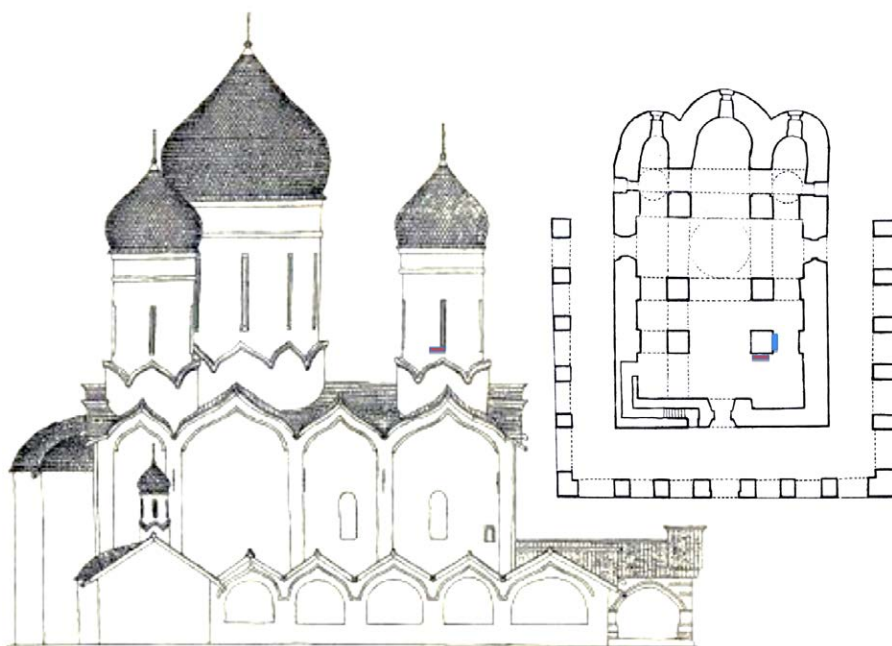
Рис. 1. Боковой фасад и план Успенского собора. Реконструкция А. Н. Милорадовича
