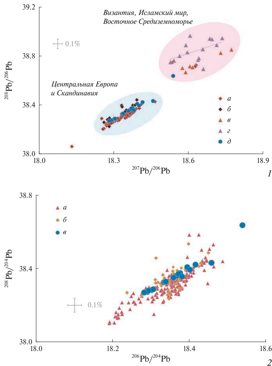
Рис. 2. Сравнение предметов из сплавов на основе меди из Суздальского Ополя/округи Муром с объектами из Центральной Европы/Южной Скандинавии и Средиземноморья (1: a – средневековая Дания; b – Германия; v – Левант; z – Эгейский бассейн; d – Ополе и Муром) и рудами (2: a – Айфель и Вестфалия (Германия); b – Девон и Корнуолл (Англия); v – Ополе и Муром).
