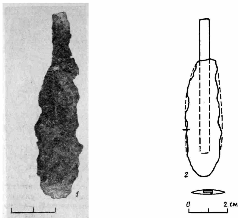
Рис. 3. 1 — биметаллический нож из кургана у с. Герасимовка; 2 — конструкция ножа
