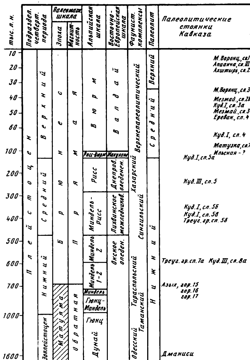
Рис. 1. Хроностратиграфическая схема палеолита Кавказа (возрастные рамки подразделений альпийской и восточноевропейских шкал по П. М. Долуханову [38])
