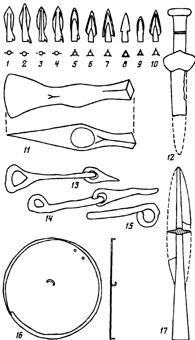
Рис. 1. Инвентарь из кург. 1 у с. Ленковцы
