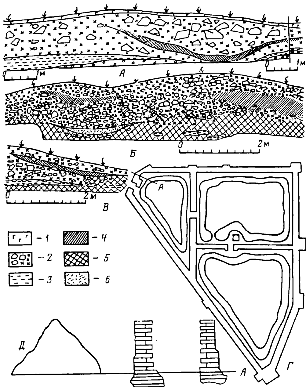
Рис. 3. Разрезы строительного мусора с делением его на два слоя серыми гумусированными прослойками и чертежи инженера Санцыперова. 1 — дерн; 2 — куски белого камня и щебень; 3 — глина; 4 — серый рыхлый слой; 5 — темно-серый культурный слой; 6 — рыба чешуя. А — разрез у привратной части; Б — разрез у юго-западной стены (внутри стен крепости); В — то же, но снаружи крепостной стены; Г — план городища, сделанный инженером Санцыперовым в 1743 г.; Д — разрез «стен» и «валов» у привратной части, сделанный Санцыперовым
