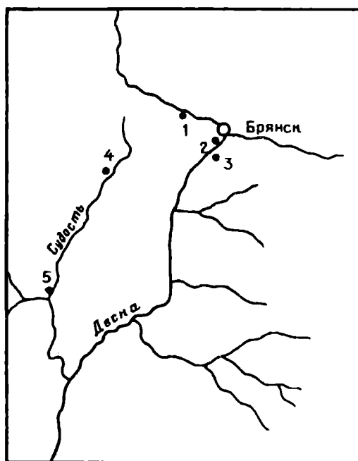
Рис. 1. Палеолитические стоянки бассейна р. Десны: 1 — Хотылево; 2 — Тимоновка; 3 — Супоново; 4 — Елисеевичи; 5 — Юдиново
