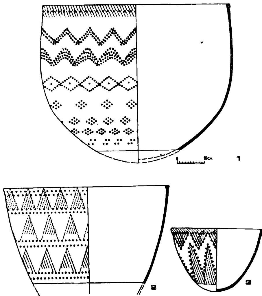
Рис. 3. Реконструкция сосудов
