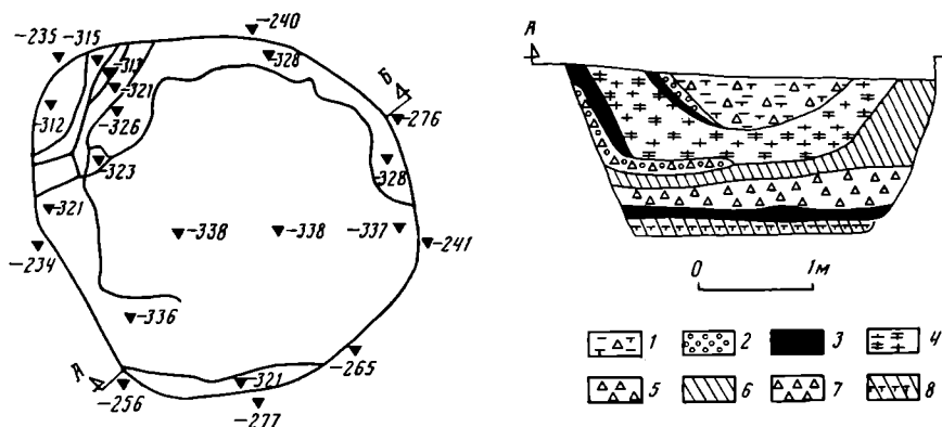
Рис. 2. План и разрез ямы. 1 — желто-серая глина со щебнем (I/1); 2 — известь (I/2); 3 — углисто-черный слой (I/3, II/2, III/2); 4 — красная, в основном обожженная глина с камнями (II/1); 5 — мелкий щебень с известью (II/3); 6 — темно-серая земля с углем (III); 7 — мелкий щебень (IV/1); 8 — желтая глина с черной землей (IV/3)
