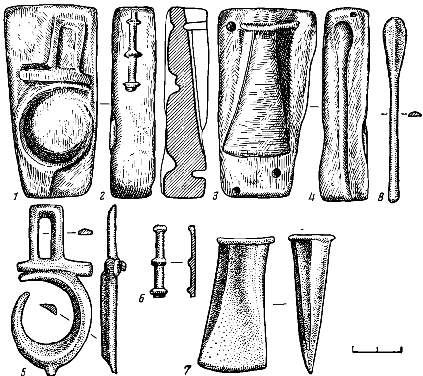
Рис. 2. Литейная форма (1—4) и предметы (5—8), реконструированные по ее негативам
