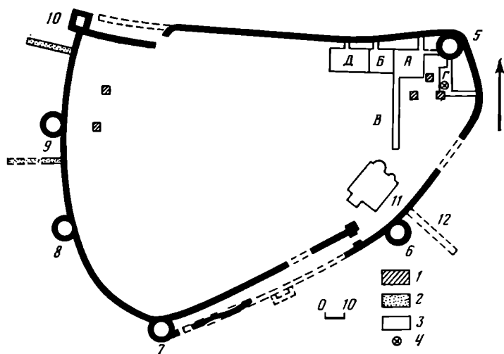
Рис. 1. Ситуационный план Изборской крепости. 1 — шурфы Н. И. Репникова (1910 г.); 2 — траншеи К. Н. Романова (1911 г.); 3 — раскопы и траншеи 1977–1980 и 1985 гг.; 4 — поруб; 5 — башня Луковка; 6 — башня Колокольная; 7 — башня Темнушка; 8 — башня Рябиновка; 9 — башня Вышка; 10 — башня Талавская; 11 — Никольский собор; 12 — подземный ход
