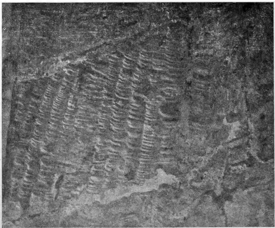
Рис. 4. Кладка западной щеки северо-восточного столба в церкви Покрова на Нерли. Обработка тесовиком с профильной заточкой
