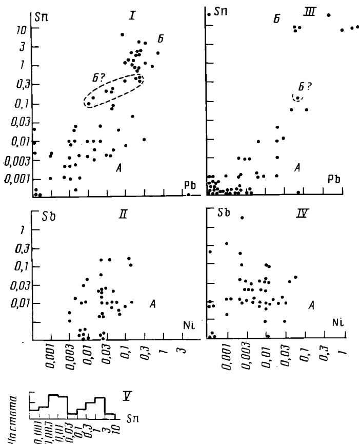
Рис. 3. Корреляционные графики и гистограмма распределения примесей в составе металла изделий могильников Гинчи (I, II, V) и Гатын-Кале (III, IV). А — мышьяковые бронзы без оловянистой литатуры; В — бронзы с оловянистой литатурой; В? — условно-оловянистые бронзы
