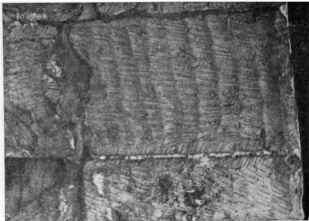
Рис. 3. Подпругная арка свода под переходом к Рождественскому собору в Боголюбове. Обработка тесовиком с профильной заточкой
