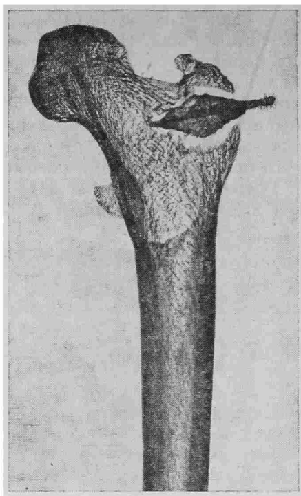
Рис. 3. Электрорентгенограмма бедренной кости с наконечником стрелы
