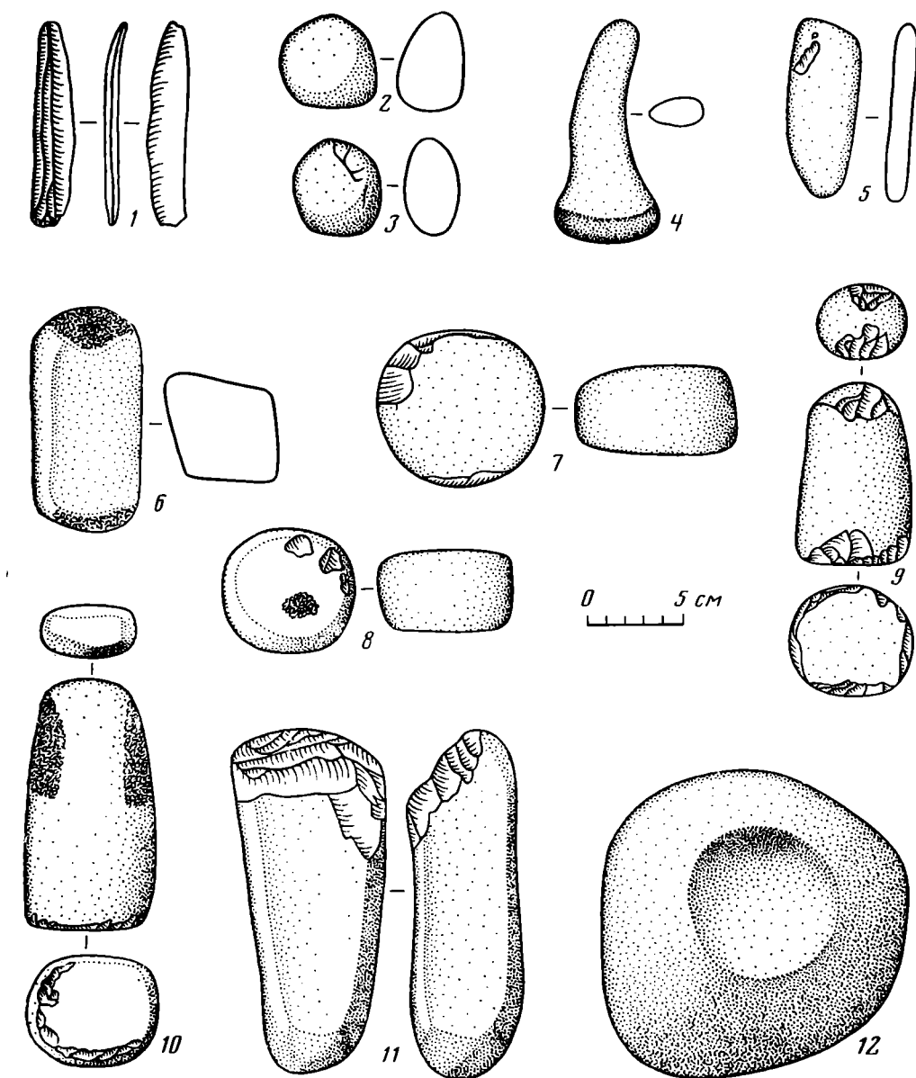
Рис. 1. Каменные орудия могильника Веселая Роща. 1, 4, 5, 7—9, 11 — группа II; 2, 3, 6, 10, 12 — группа III
