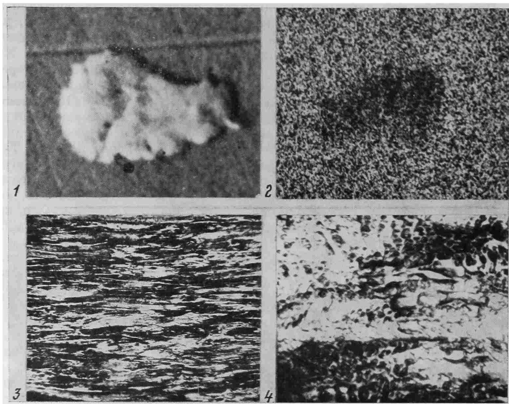
Рис. 3. Фотографии микроструктуры медной сердцевины шила. 1, 2 — электронно-микроскопическое изображение (ув. 10 000); 3, 4 — металлографическое изображение (3 — ув. 130, 4 — ув. 400)
