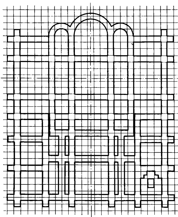
Рис. 5. Реконструкция плана фундаментов Десятинной церкви
