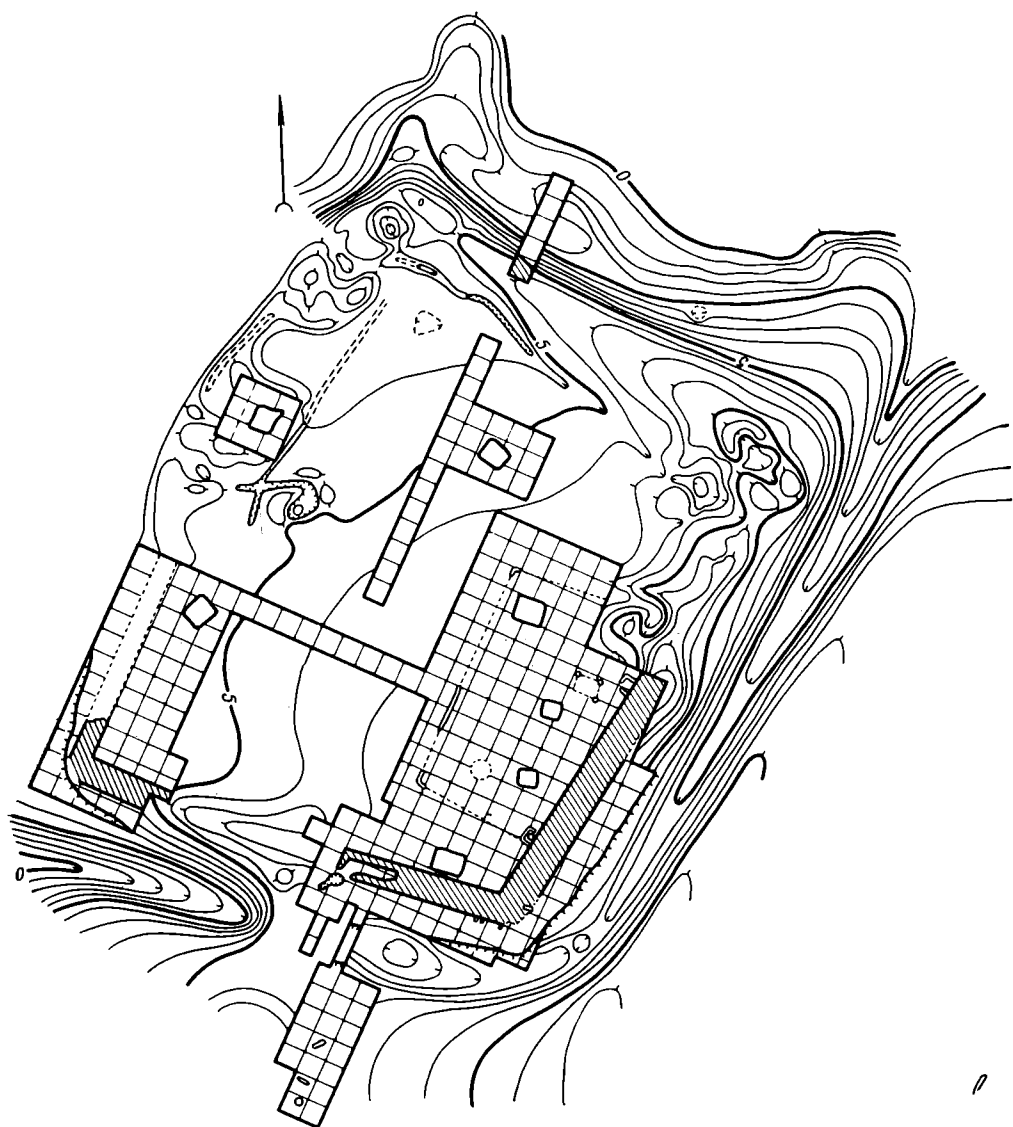
Рис. 1. План Маядковской крепости
