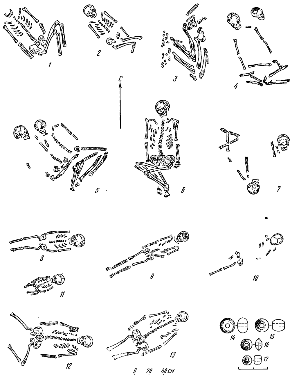
Рис. 4. Дрони́хинский моги́льник: 1 — погр. 1; 2 — погр. 4; 3 — погр. 12; 4 — погр. 18; 5 — погр. 19; 6 — погр. 20; 7 — погр. 21; 8 — погр. 5; 9 — погр. 7; 10 — погр. 8; 11 — погр. 9; 12 — погр. 11; 13 — погр. 13; 14—17 — пастовые бусы из погр. 7
