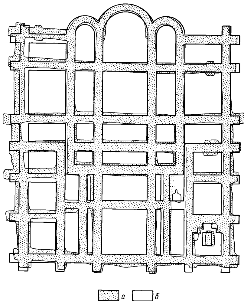
Рис. 6. Сопоставление сохранившихся и реконструируемых планов фундаментов Десятинной церкви: а — план фундаментов, вскрытых археологическими раскопками; б — реконструируемый план фундаментов
