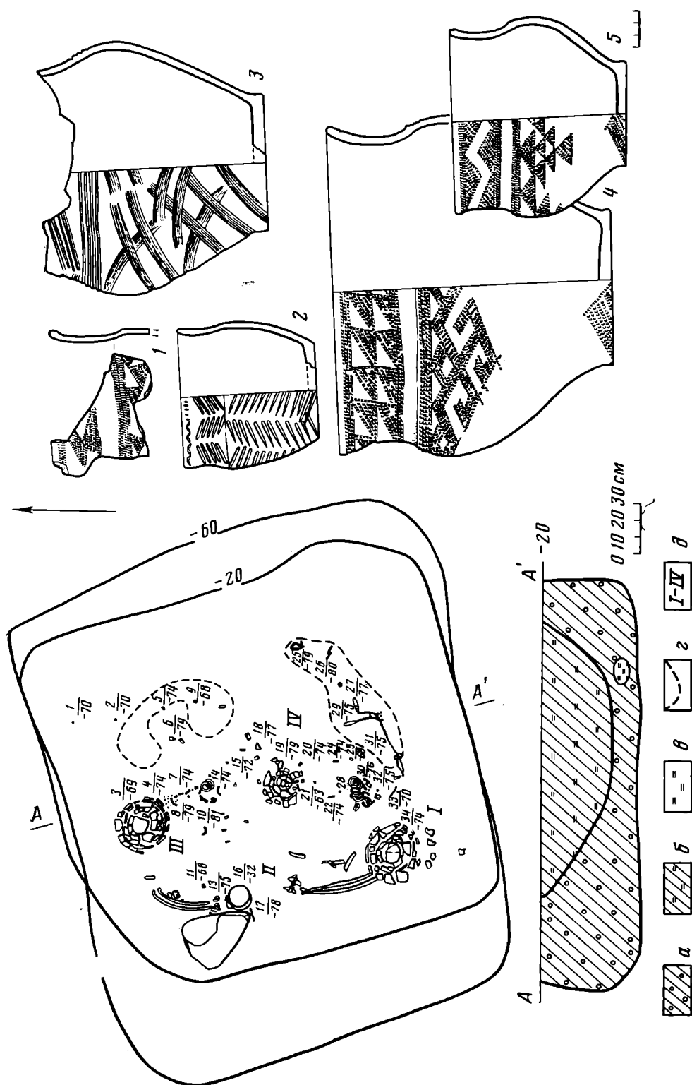
Рис. 2. Могильник Ку- левчи VI. Курган 3, яма 2, план и разрез. 1, 3—5 — керамика из ямы; 2; 2 — сосуд из ямы 1; а — серый грунт с гра- висем; б — темно-серый грунт с глиной, песком; в — глина; г — границы скопления калыциниро- ванных костей; д — со- суды
