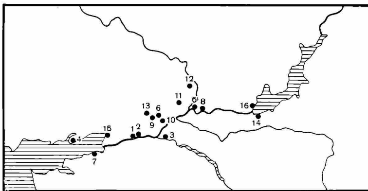
Рис. 5. Памятники Нижнего Подонья. 1 — Аксай, 2 — Алптуб, 3 — у ст. Багаевской, 4 — Беглицкая коса, 5 — Бронницкая переправа, 6 — Заплавская, 7 — Комаровка, 8 — Константиновка, 9 — Красюковская, 10 — Кривянская, 11 — Крымский, 12 — Нижнекундрючевская, 13 — Новочеркасск, 14 — Саркел, 15 — Недвиговка, 16 — Цимлянск
