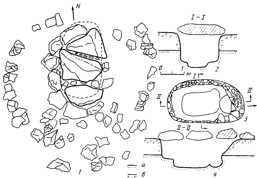
Рис. 4. Кургan 23: 1—4 — планы и разрезы; а — туфовая скала; б — галька
