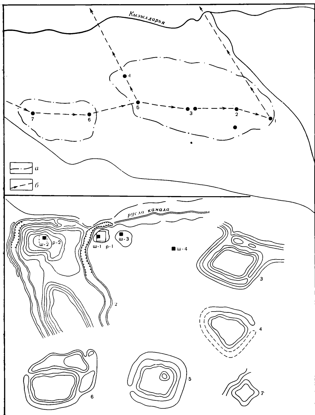
Рис. 1. Схема расположения и планы поселений Кайрагачского и Гульдаринского культурно-хозяйственных районов. 1 — Кайрагачтепе; 2 — Даратепе; 3 — Туртбурчактепе; 4 — Самантепе; 5 — Кузатепе; 6 — Курганча; 7 — Бешкутантепе а — границы оазисов; б — древние пути
