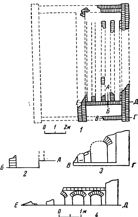
Рис. 54. Обжигательная печь одного из кирпичных заводов под Звенигородом
