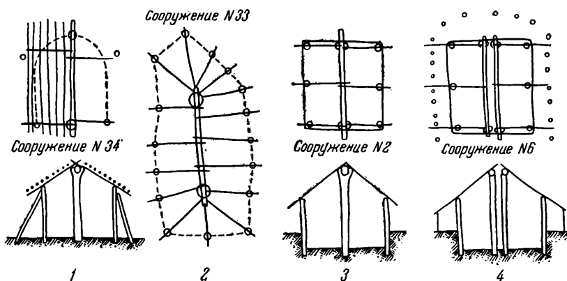
Рис. 13. Тетеревка I. Конструктивные схемы построек
