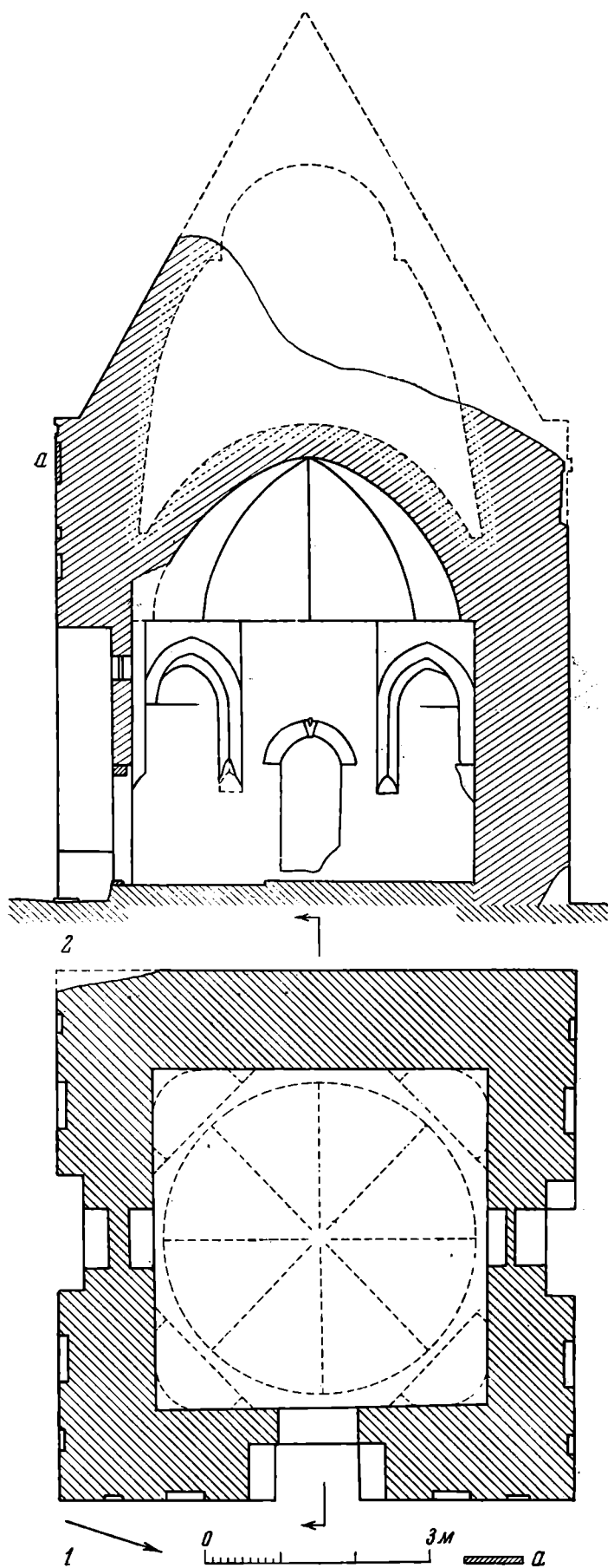
Рис. 22. Мавзолей Бабаджи Хатун. План (1) и разрез (2). а — наравды с арабской надписью.
