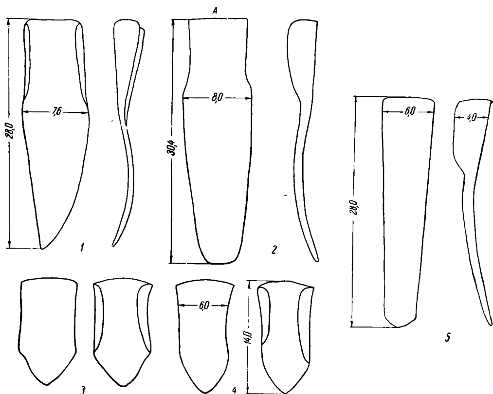
Рис. 5. Типы болгарских сошников (1—4) и древнерусский сошник из Новгорода (5).
