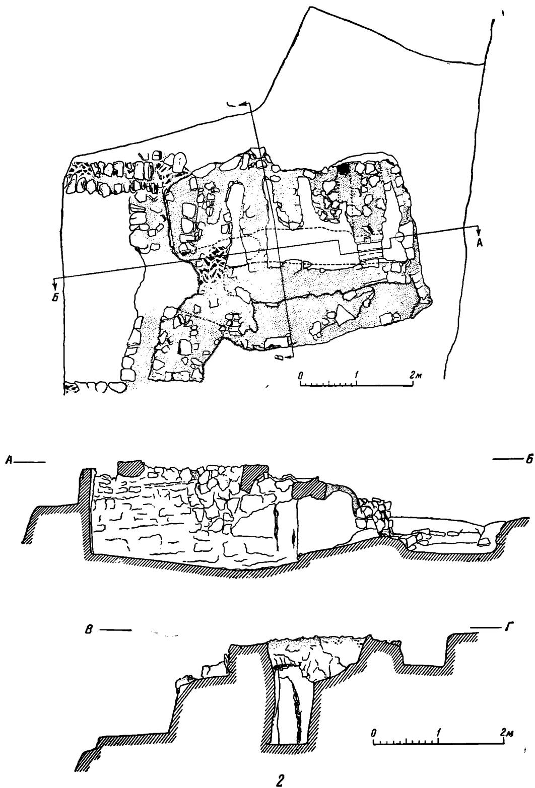
Рис. 73. План и разрезы гончарной печи № 5.
