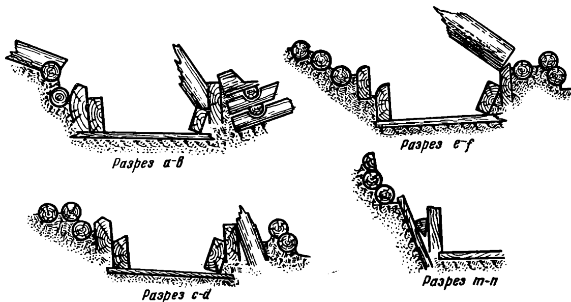
Рис. 13. Сечения ряжей
