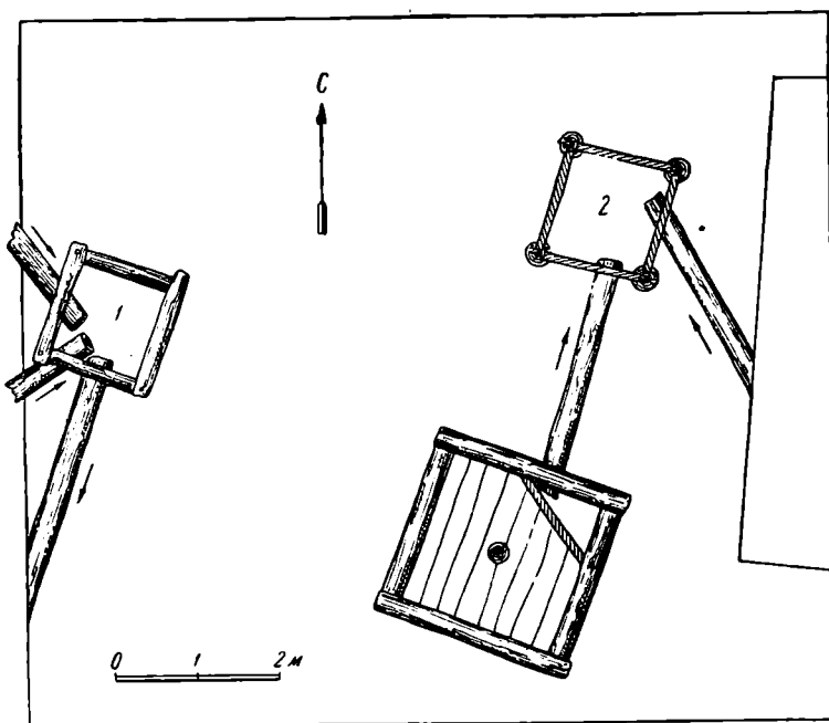
Рис. 13. Водоотводные сооружения XIII XIV вв. на Софийской стороне.
