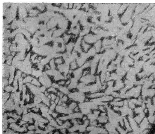
Рис. 8. Микроструктура
