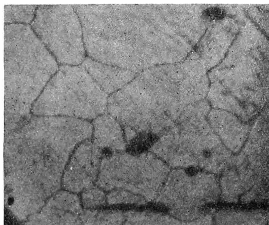
Рис. 7. Микроструктура
