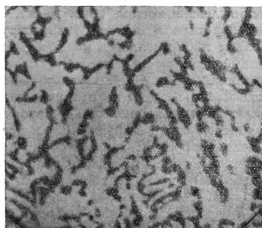
Рис. 8. Микроструктура
