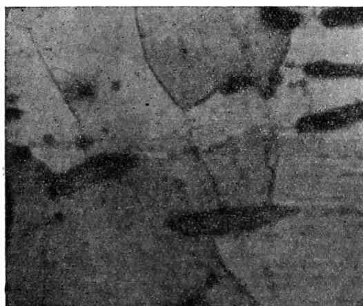
Рис. 7. Микроструктура
