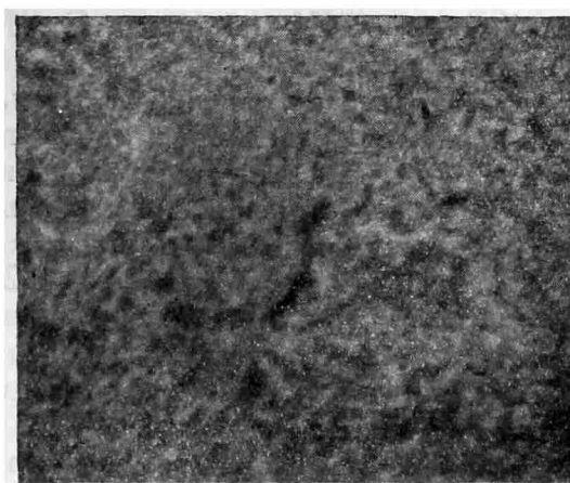
Рис. 9. Микроструктура
