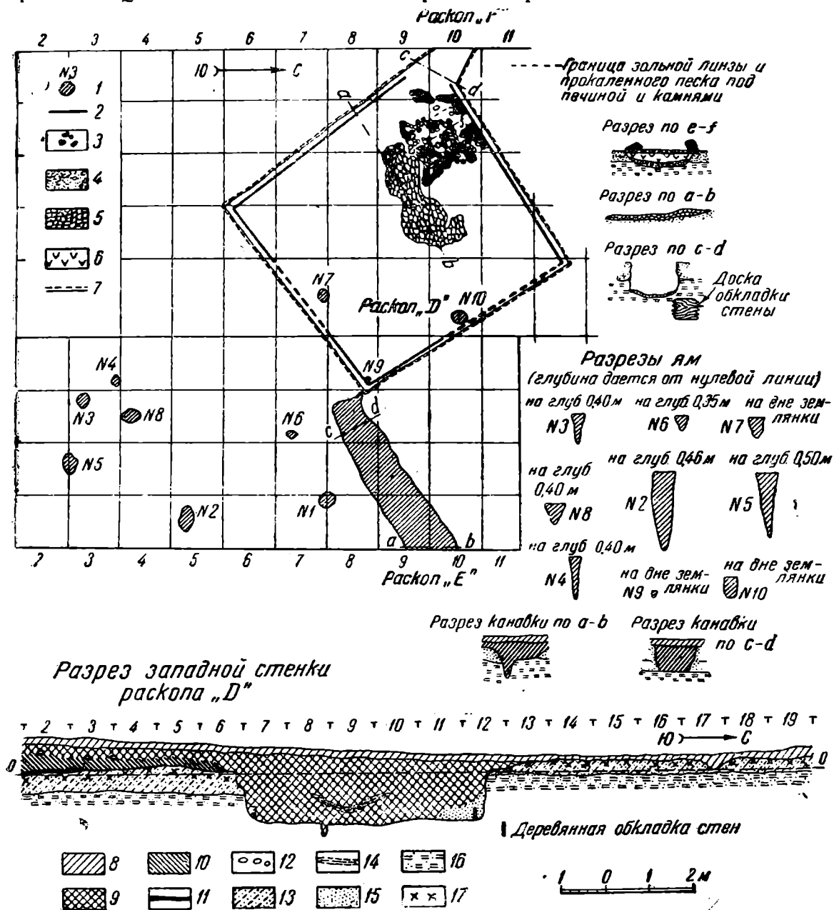
Рис. 22. Планы и разрезы сооружений из раскопок 1946 г. Городище «Песочный Ров» 1 — ямы; 2 — доска; 3 — камни; 4 — обожженный песок; 5 — печина; 6 — зола; 7 — граница землянки; 8 — пахотный слой; 9 — культурный слой; 10 — культурный слой I; 11 — чернозем; 12 — обломки пещины; 13 — подзол-беловатая супесь; 14 — кострище; 15 — песок; 16 — плотный суглинок с ортзан-дами; 17 — кремневые поделки
