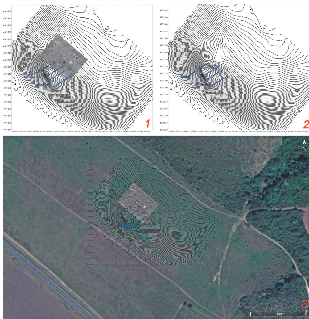
Рис. 3. Пос. Куматырь: 1 – магнитная карта на фоне топосъемки; 2 – расположение выявленных объектов на топосъемке; 3 – магнитная карта на фоне топосъемки и космического снимка
