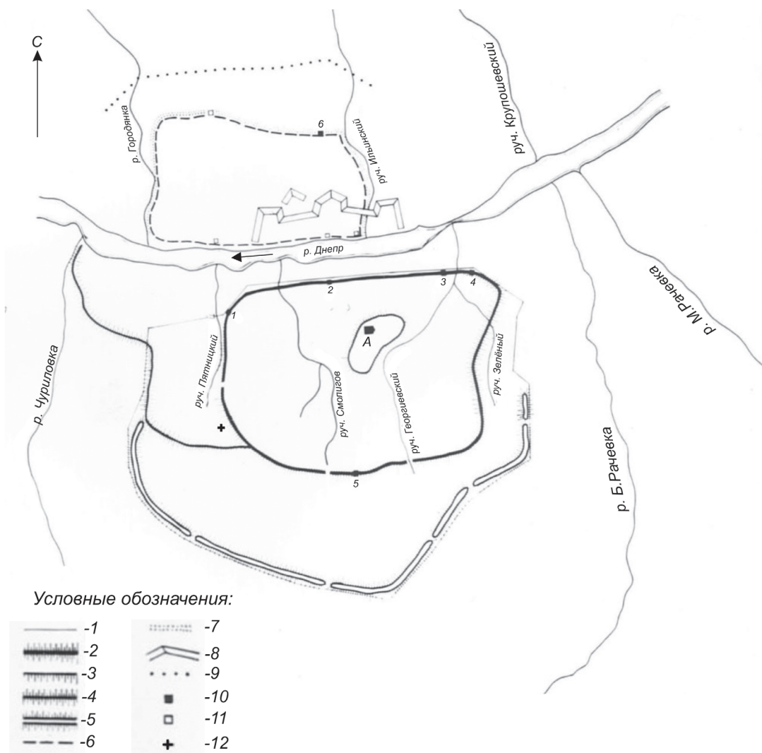
Рис. 21. Оборонительные сооружения г. Смоленска XII – начала XVIII вв.
