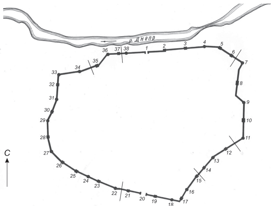
Рис. 43. План крепости (1596–1602) с перечнем башен по росписи М. Шеина 1609 г.
