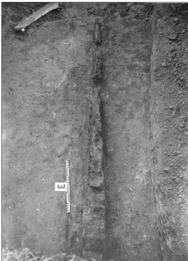
Рис. 32. Земляной вал XVI в. Полости от деревянных внутриральных конструкций. Раскопки 1981 г.
