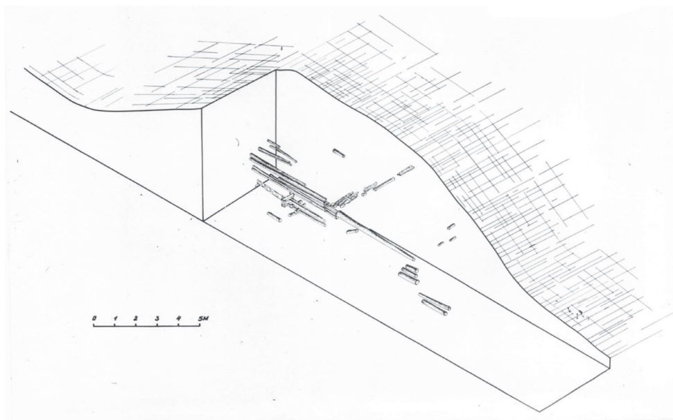
Рис. 34. Вал «Нового большого города» (XVI в.). Расположение остатков внутривальных конструкций. Раскопки в парке «Лопатинский сад», 1978 и 1981 гг. Аксонометрия
