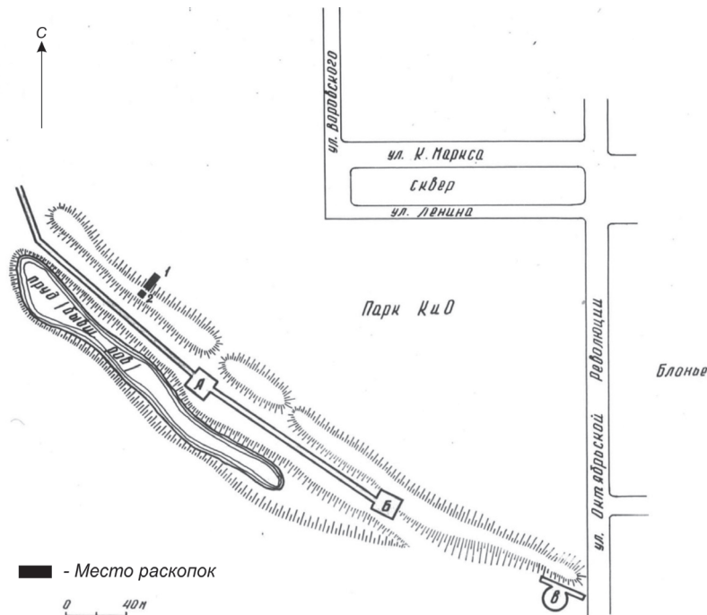
Рис. 29. Вал «Большого нового города» (XVI в.). План с нанесением места раскопок 1978 и 1981 гг. 1. Раскоп 1976 г.; 2. Раскоп 1981 г. А – Копытецкие ворота; Б – башня Бублейка; В – башня Громовая.
