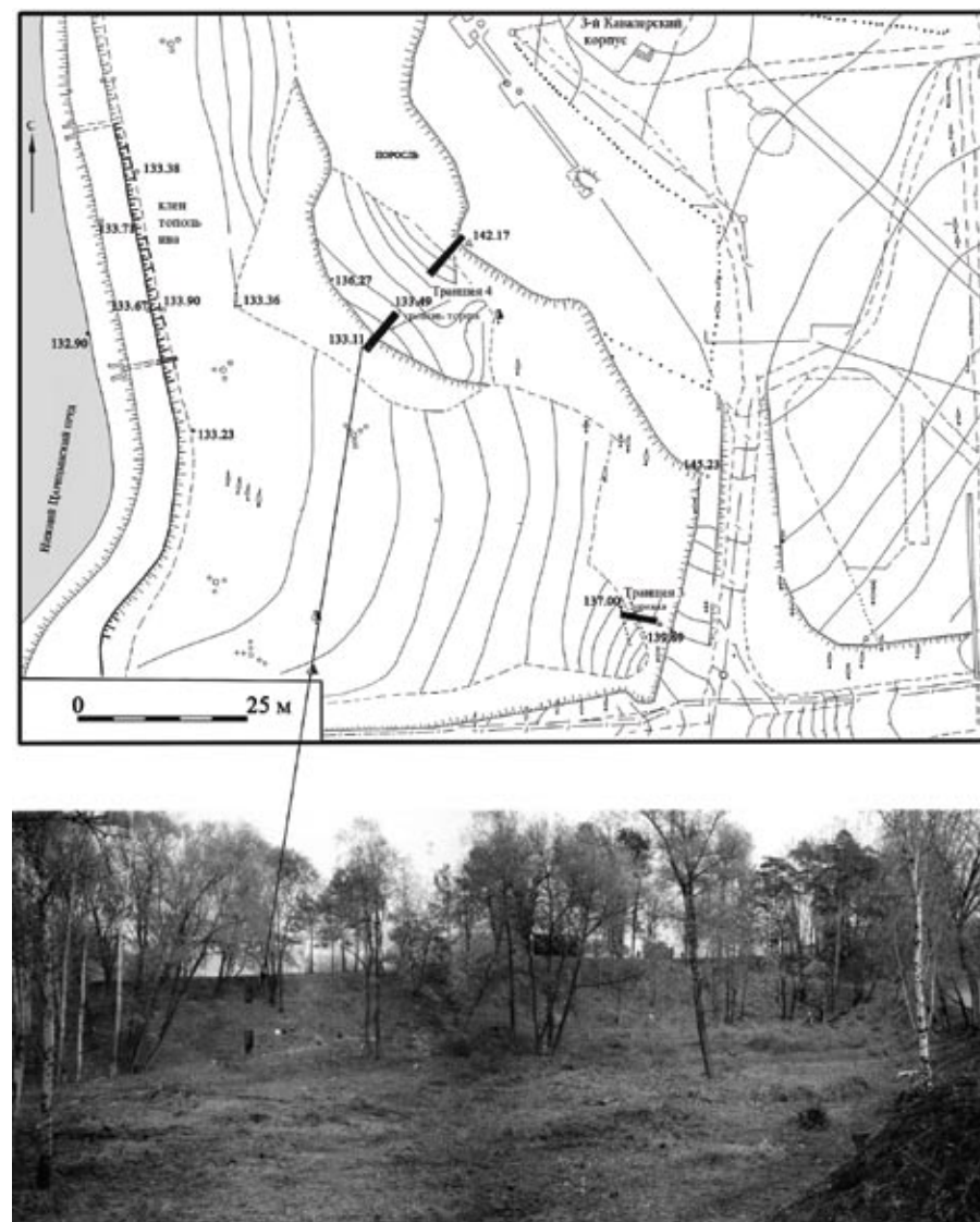
Рис. 26. План и фотография участка работ на берегу Нижнего Царицынского пруда под Третьим Кавалерским корпусом, траншеи № 3 и № 4
