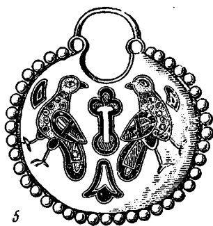
Рис. 94. Процесс изготовления колта с перегородчатой эмалью: 1 — про- резная матрица для тиснения золотых листов; 2 — тиснение золотого листа; 3 — напаяны перегородки для разных цветов эмали; 4 — увели- ченная деталь колта (в перспективе); 5 — перегородки заполнены эмалью; 6 — вид колта сбоку.
