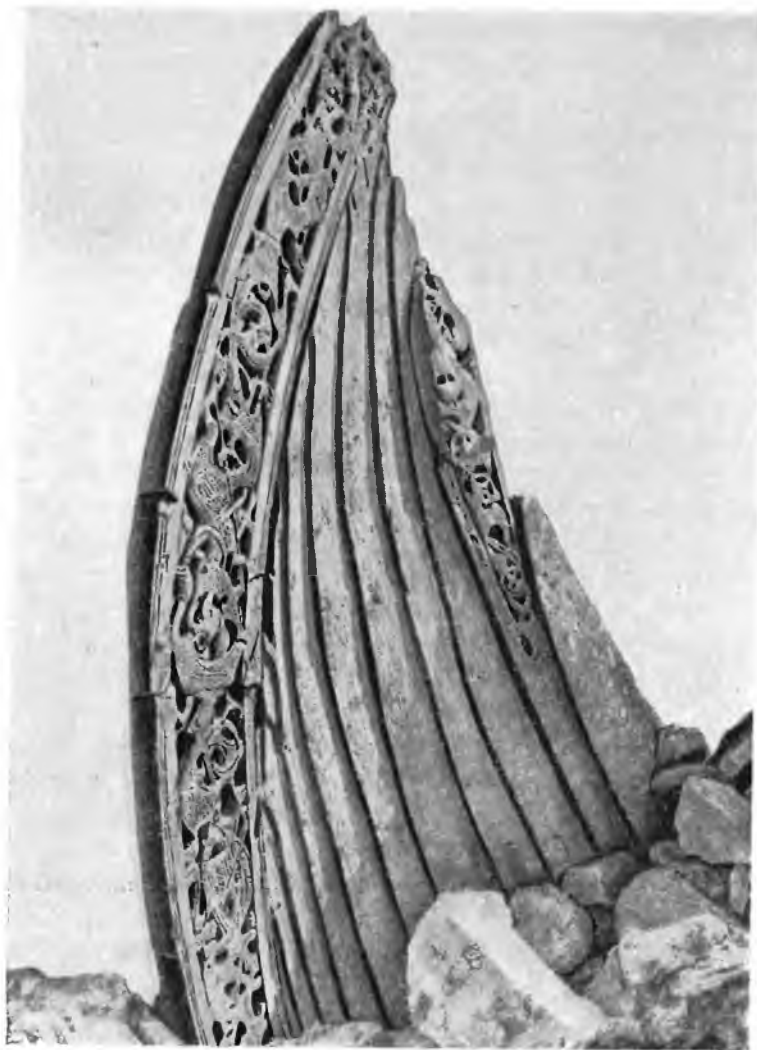
Рис. 189. Носовая часть Озебергского корабля
