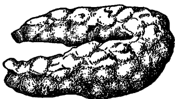
Рис. 44. Крица, найденная в Вышгороде (раскопки Б. А. Рыбакова).
