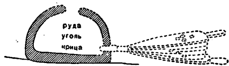
Рис. 42. Домница («сыродутный горн») с Лабенского городища. Разрез.
