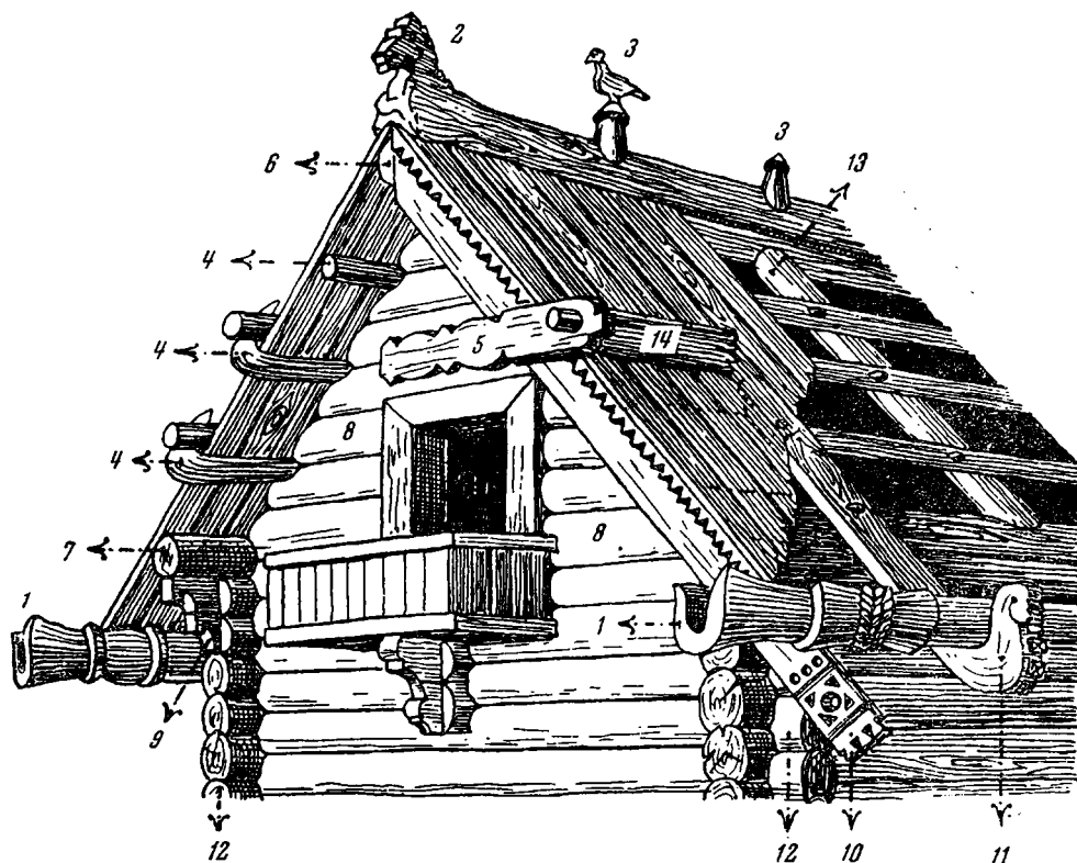
Рис. 130. Схема устройства кровли (по М. В. Красовскому). 1 — жолоб; 2 — охлупень; 3 — стамик; 4 — слега; 5 — огниво; 6 — князевая слега («кнес»); 7 — повальная слега; 8 — самец; 9 — повал; 10 — причелина; 11 — журица; 12 — пропуск; 13 — бык; 14 — гнет.
