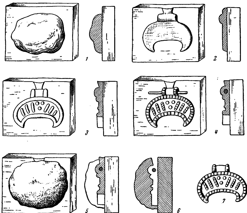
Рис. 55. Стадии изготовления вшей по восковой модели: 1 — на огнеупорную поверхность накладывается слой воска; 2 — воск обрезан по форме будущей лунницы; 3 — на плоскость восковой модели наложены валики из воска; 4 — острием на воске нанесен орнамент, в ушко продет стержень; восковая модель готова; 5 — восковая модель залита жидкой глиной; 6 — воск вытоплен, на его место налит металл; 7 — готовая лунница.
