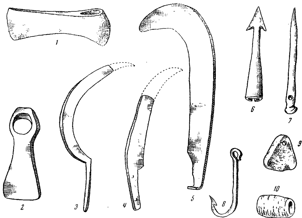
Рис. 24. Орудия сельского хозяйства и промыслов VIII—X вв.: 1 — топор; 2 — мотыга; 3—5 — серпы; 6 — наконечник копья; 7 — костяная игла для вязания сетей; 8 — рыболовный крючок; 9—10 — грузила для сетей.
