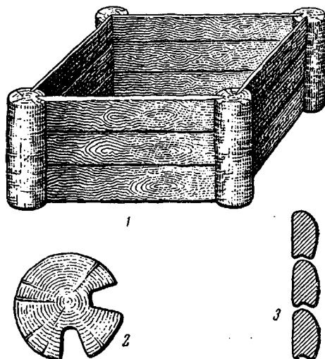
Рис. 102. Кожевенный чан: 1 — общий вид; 2—3 — детали (Новгород. Раскопки А. В. Арпиховского).
