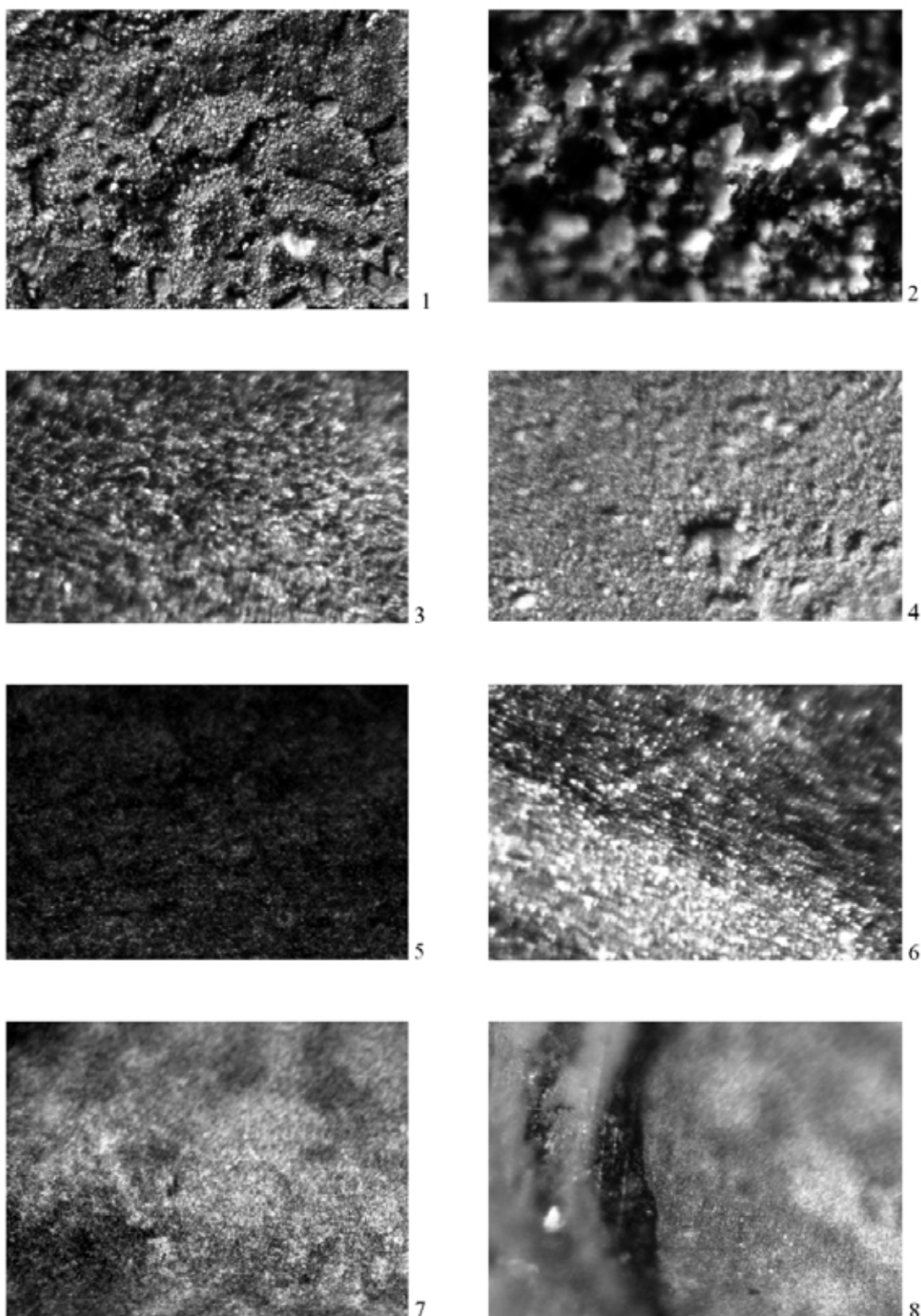
Рис 1. Микроструктуры перстней со средневековых памятников Пермского Предуралья.
