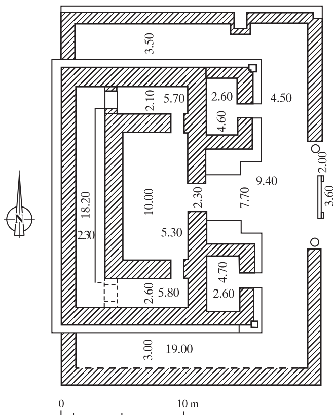
Рис. 5. Дильберджин. Храм Диоскуров. План.
