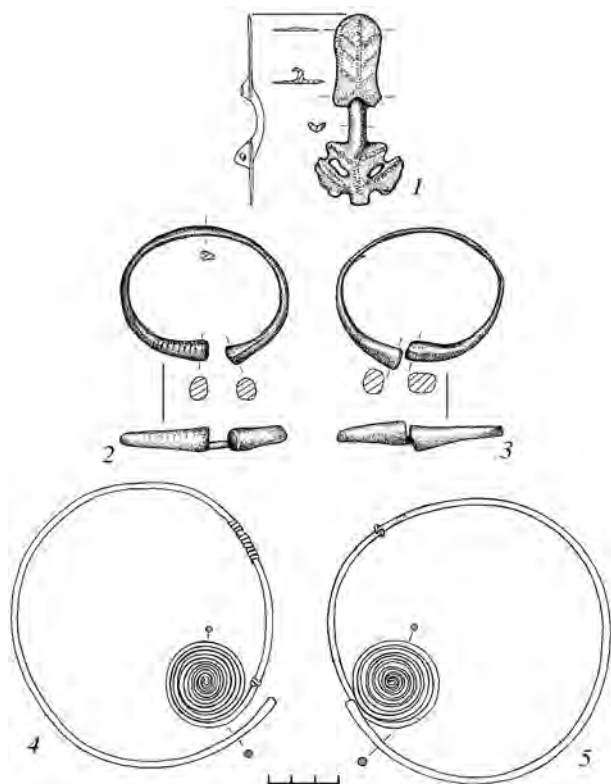
Рис. 2. Куриловский клад. 1 – фибула антропоморфная; 2, 3 – браслеты; 4, 5 – височные кольца. Сплав на медной основе.
