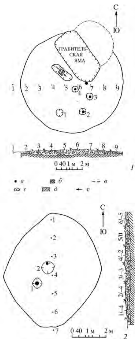
Рис. 3. Планы и профили раскопанных курганов в урочище Кезек-Хурээ: 1 – курган 1; 2 – курган 2; а – деревянные столбы, б – стела, в – граница выброса, г – камни, д – материк, е – расположение надписей (по: Кызласов Л.Р., 1960в. Рис. 172, 173).
