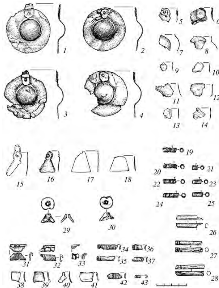
Рис. 4. Куриловский клад. 1–14 – умбовидные подвески; 15–18 – трапециевидные подвески; 19–25 – спиральные пронизы; 26–28 – трубчатые пронизы; 29, 30 – ворворки; 31–43 – фрагменты предметов неясного облика. 1–28 – сплав на медной основе; 29–43 – свинцово-оловянный сплав.
