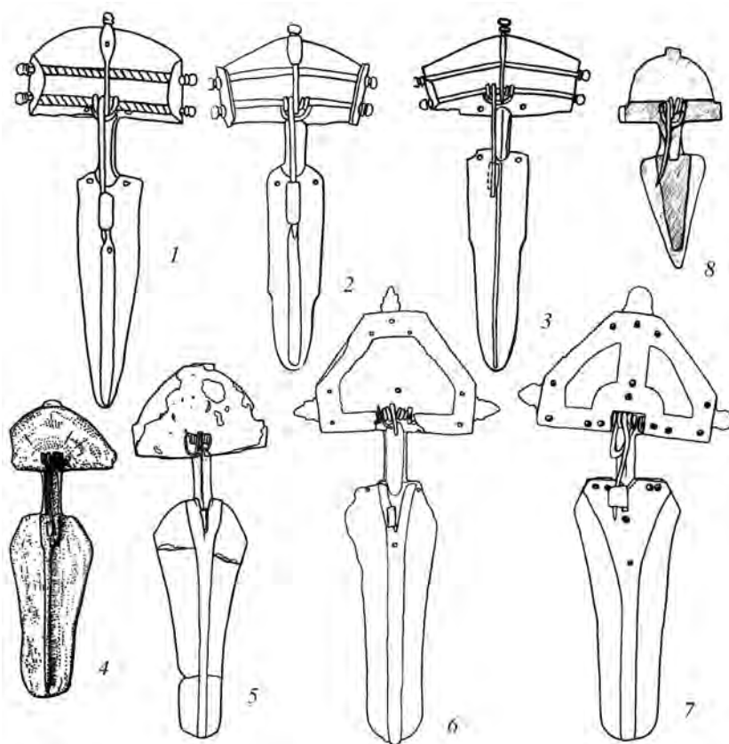
Рис. 4. Разновидности каркаса двупластинчатых фибул Крыма и Северо-Восточного Причерноморья. 1–3 – могильник на р. Дюрсо (по: Дмитриев, 1982); 4 – Лучистое (по: Айбабин, 1994); 5–8 – Суук-Су (8 – по: Айбабин, 1990).
