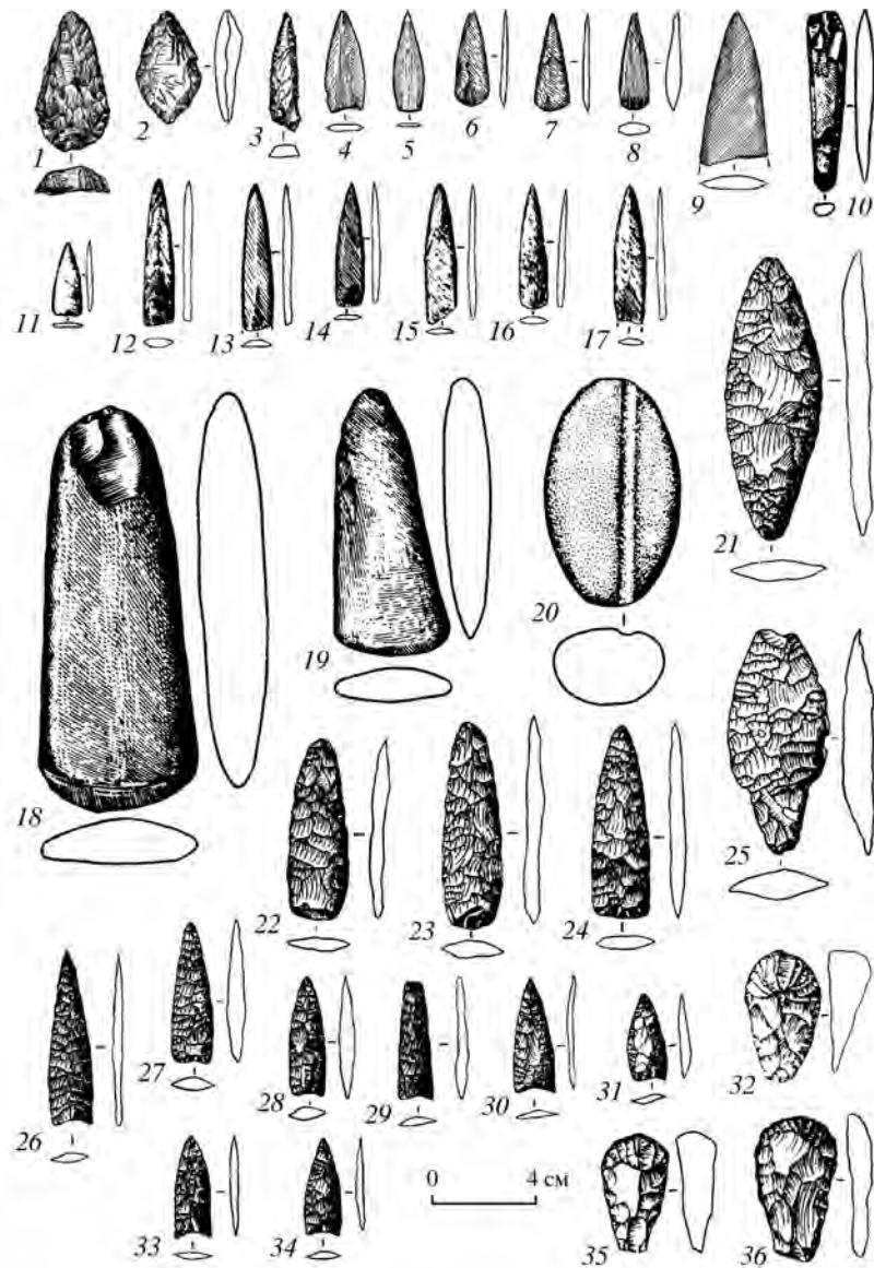
Рис. 6. Каменный инвентарь, соответствующий керамике сергеевского типа: 1–9 – Сергеевка-1 (по: Батаршев, Попов, 2008); 10–36 – Чертовы Ворота (по: Неолит юга..., 1991).
