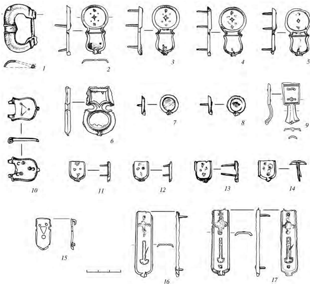
Рис. 6. Куриловский клад. Детали ременной гарнитуры. Сплав на медной основе.
