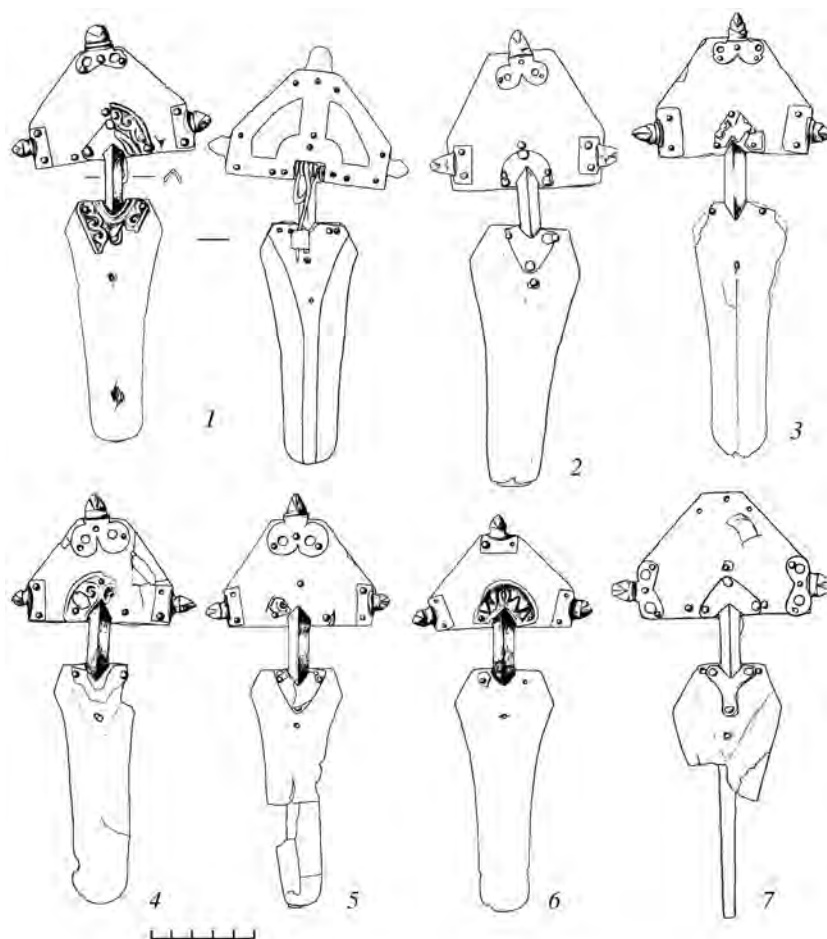
Рис. 3. Большие двухпластинчатые фибулы с накладками из Южного Крыма. 1 – Суук-Су, погребение 89; 2 – Суук-Су, погребение 46-II (по: Амброз, 1966); 3 – Суук-Су, погребение 56-V; 4, 5 – Суук-Су, погребение 56-III; 6 – Суук-Су, погребение 91; 7 – Артек, разрушенное погребение.
