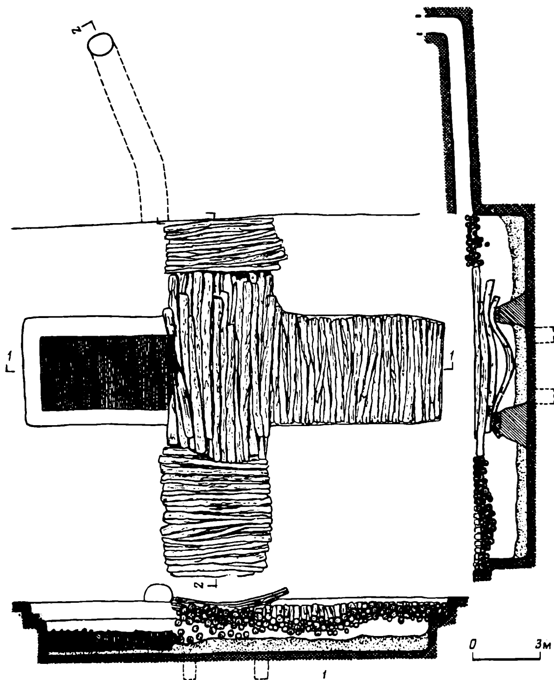
Рис. 1. План могильной камеры Сарычобанского кургана. 1 — план и разрез перекрестия; 2 — план и разрез камеры после очистки
