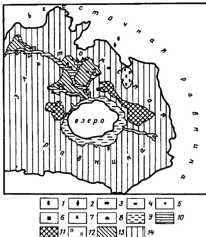
Рис. 1. Геоморфологическое районирование Эльтонской равнины. Объекты исследования: 1 — Вишневка-82; 2 — Вишневка-78; 3 — Ченин-80; 4 — Эльтон-84; 5 — Венгилевка-82; 6 — Эльтон-83; 7 — Красная Деревня-81; 8 — Приозерное-85. Геоморфологические районы: 9 — озерные террасы; 10 — долины рек и балки; 11 — солянокупольные поднятия; 12 — лиманные понижения; 13 — речные и балочные водоразделы; 14 — равнинные степные участки
