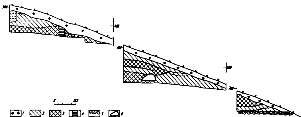
Рис. 1. Телль Хазна I. Разрез по северной бровке траншеи. 1 — верхний мешаный слой; 2 — слой серый глинистый; 3 — слой желто-коричневый глинистый; 4 — кладка; 5 — материк; 6 — кротовины
