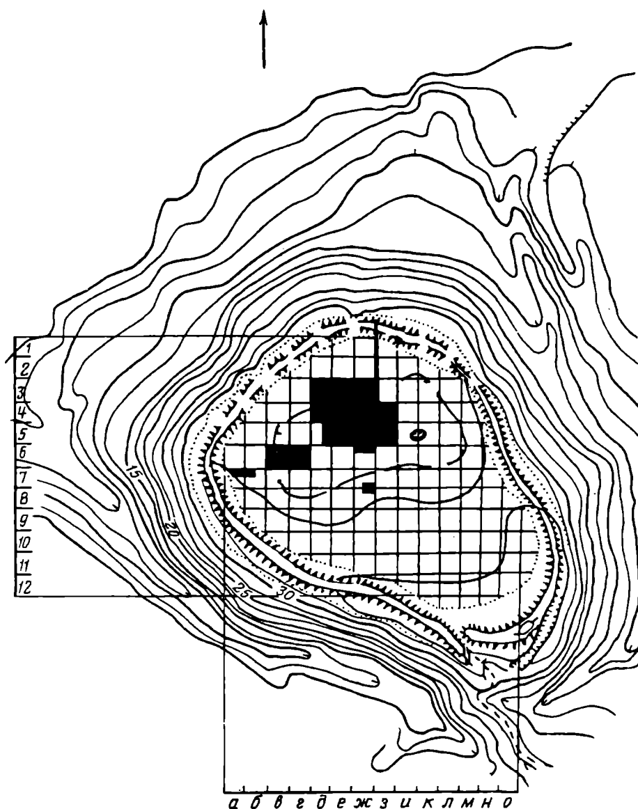
Рис. 1. Мстиславский детинец, план. Сплошные горизонталы проведены через 2 м
