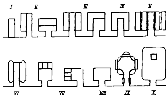
Рис. 2. Основные «архитектурные» типы подземных сооружений (по А. Б. Авагяну)
