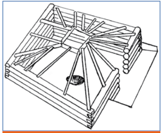
Каркасно-столбовая конструкция одинцовского жилища с поселения Сошниково-1. Реконструкция А.А. Казакова, рисунок О.А. Семибратовой
