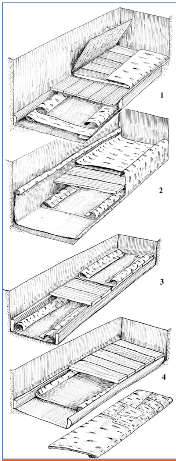
Реконструкция внутримогильных конструкций на памятнике Усть-Алейка-Клуб (по: [Тишкин, 2009])
